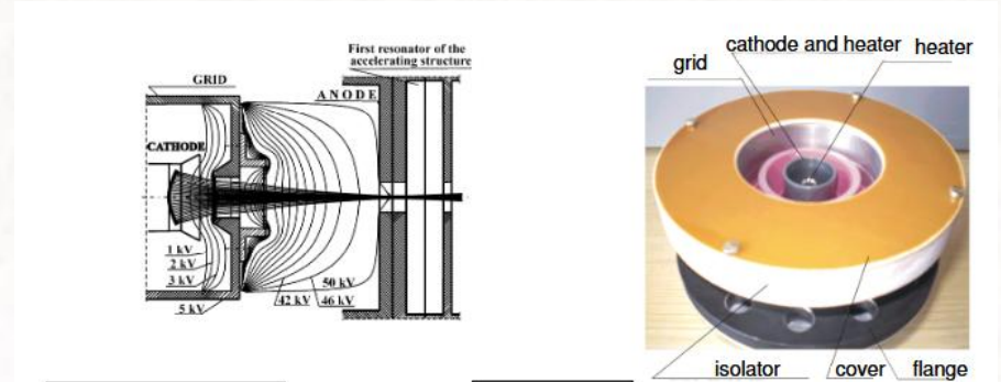
Sumber Elektron LINAC Medis
