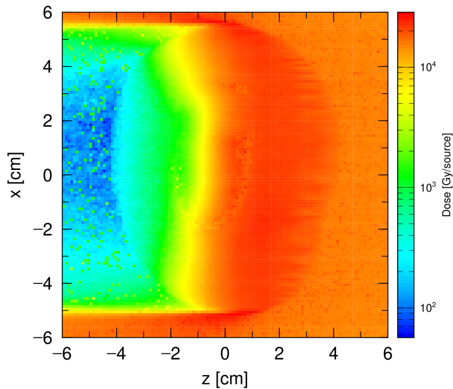
Sumber Elektron 10 MeV
