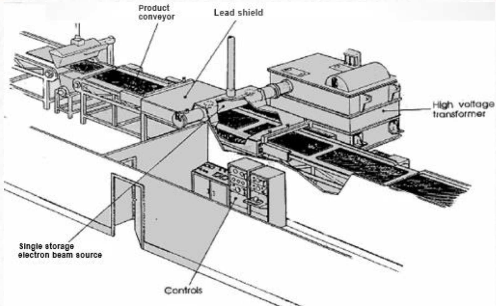
Gambar 1. Iradiator elektron/ion dengan energi dibawah 0,5 MeV
